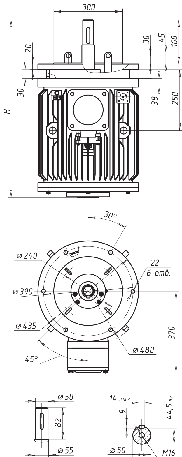
Рисунок 10. ВАСОУ-9 (-13, -15, -18,5) -12 (Монтажное исполнение IM 3031)
