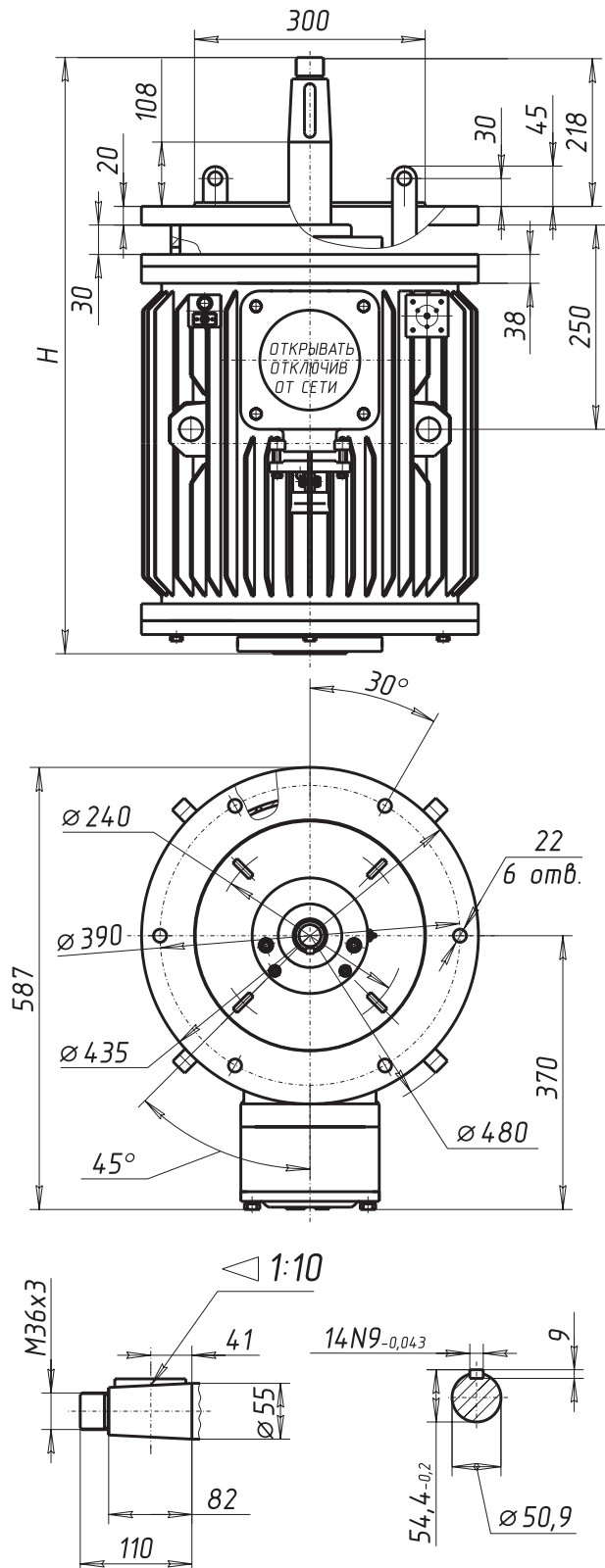
Рисунок 12. ВАСОУ-9 (-13, -15, -18,5) -12 (Монтажное исполнение IM 3033)
