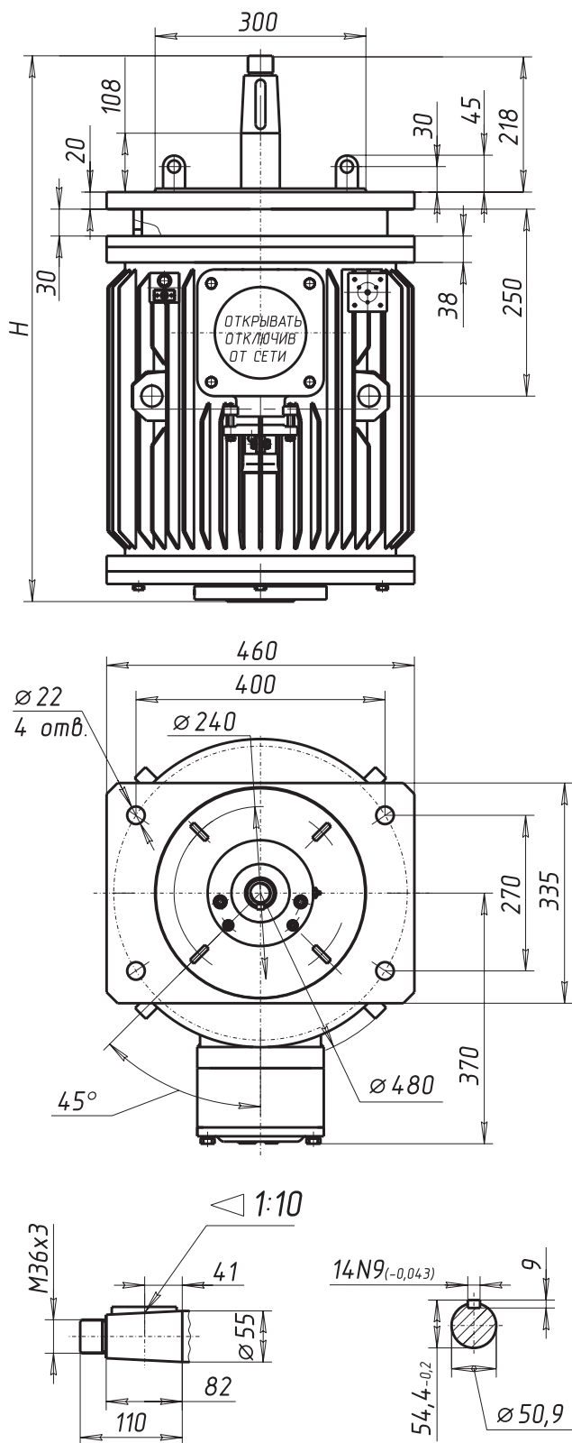
Рисунок 11. ВАСОУ-9 (-13, -15, -18,5) -12 (Монтажное исполнение IM 3033) (с квадратным фланцем)
